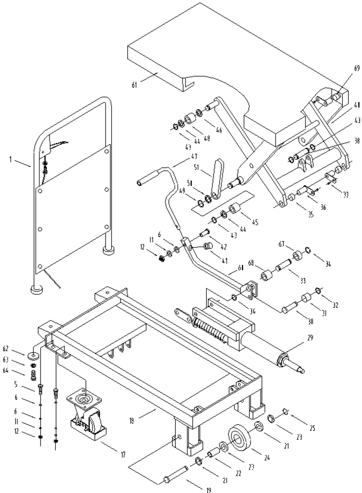
Abbildung 2 Rahmen
