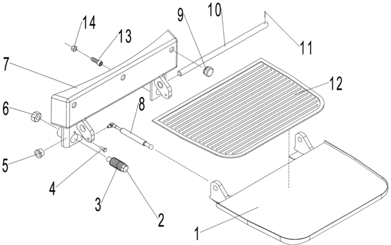
Abbildung 16 Expl. Mitfahrerplatte
