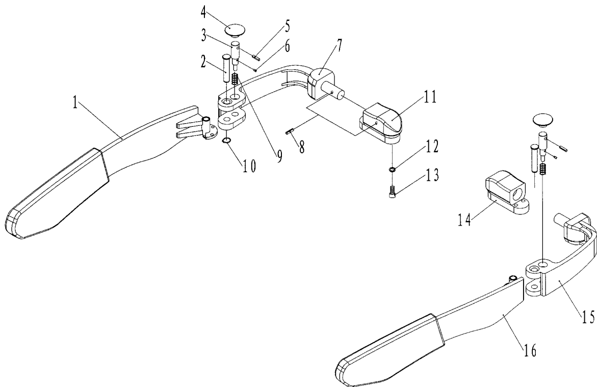
Abbildung 18 Expl. Seitenarme B
