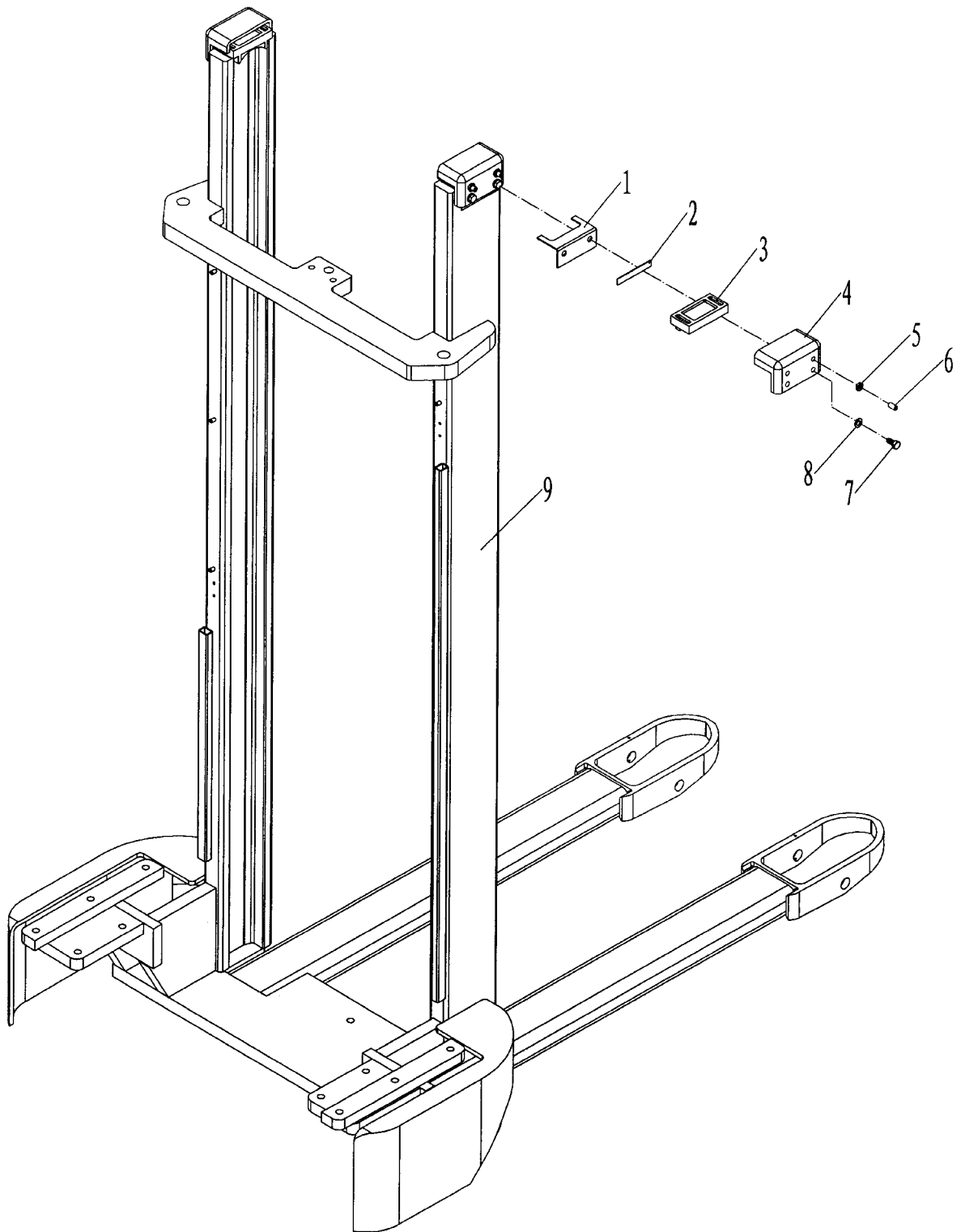
Abbildung 13 Expl. Mast / Rahmen
