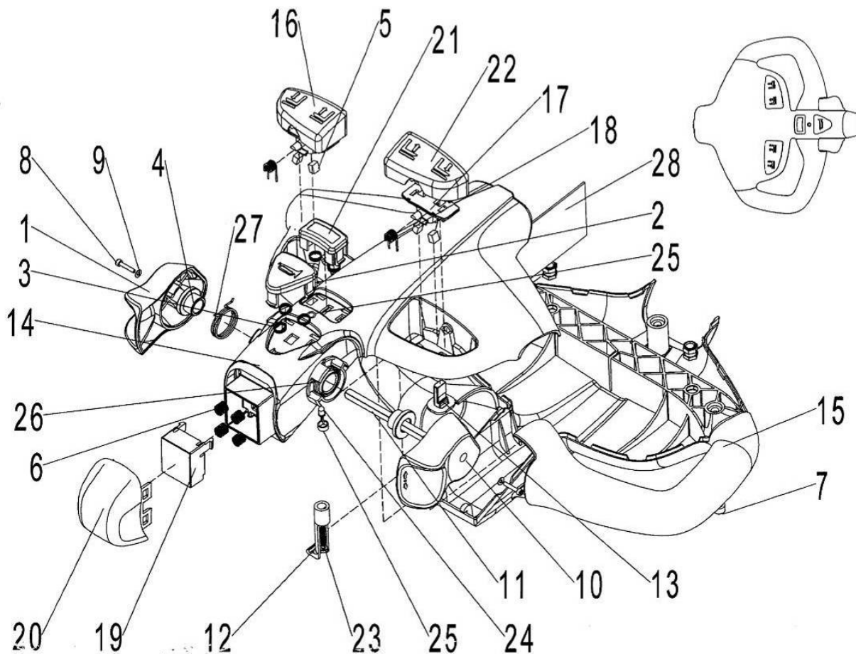
Abbildung 20 Expl. Deichselkopf
