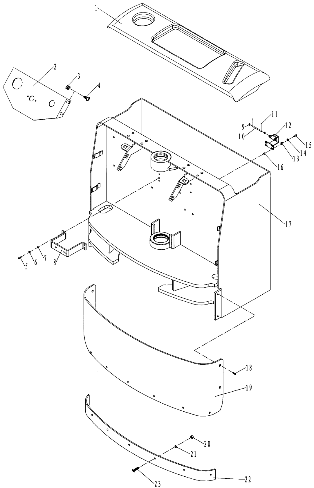
Abbildung 2 Expl. Batteriebox
