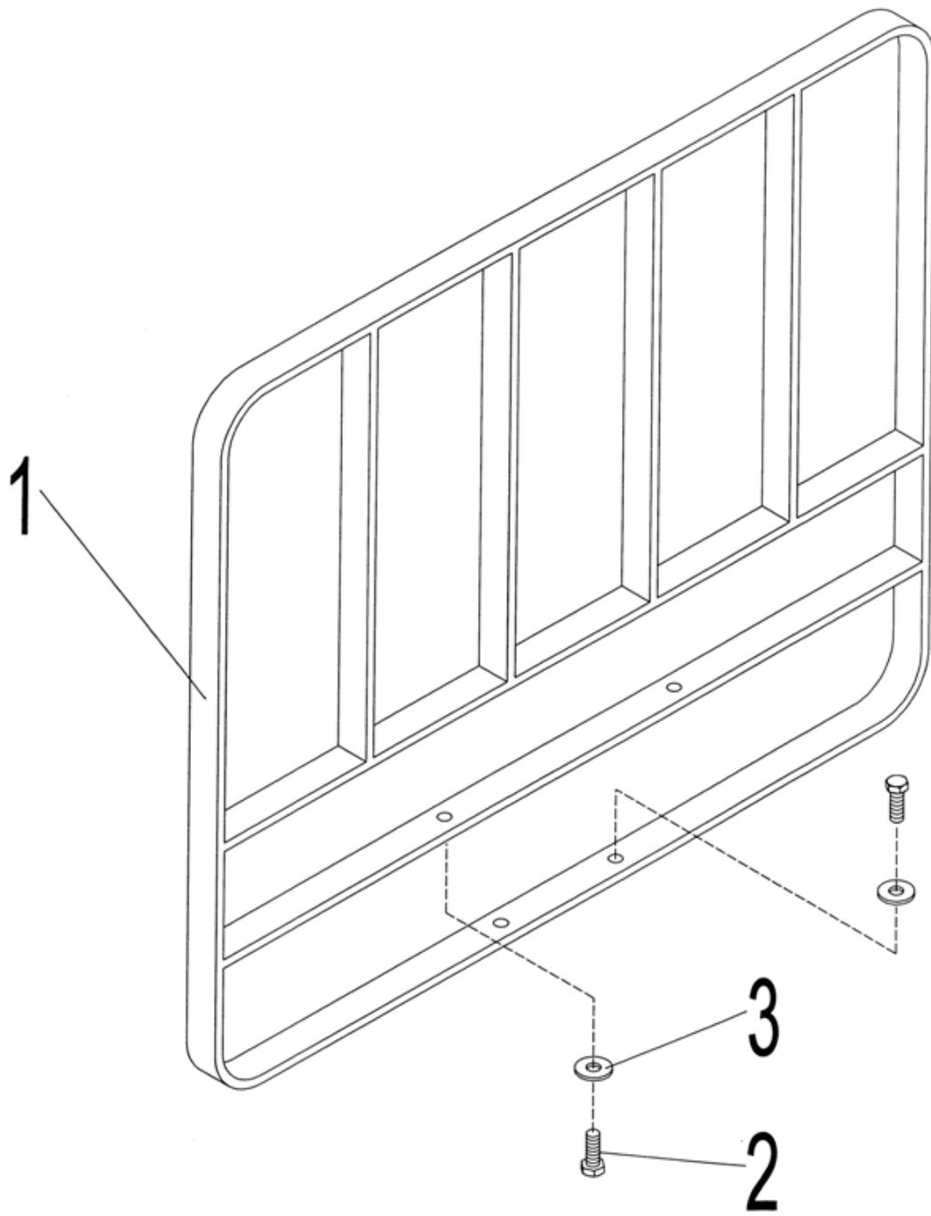
Abbildung 19 Expl. Lastschutzgitter
