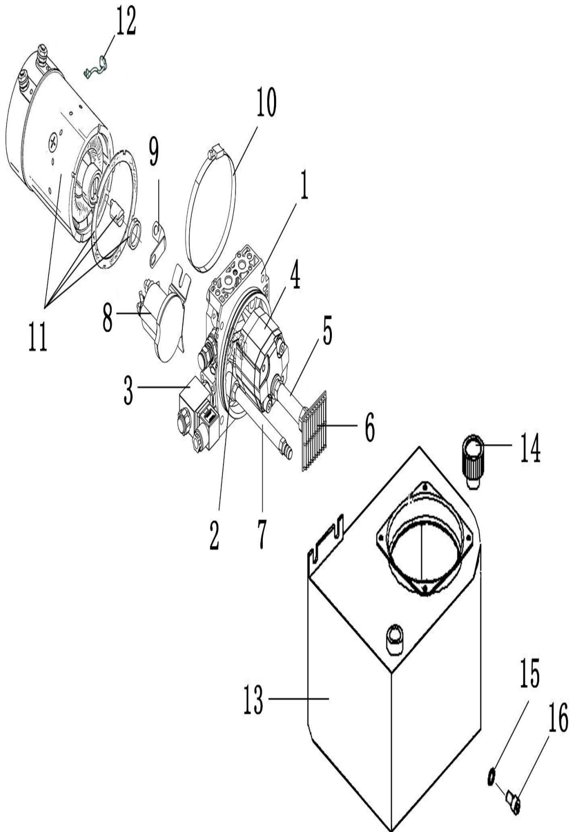
Abbildung 12 Expl. Hydraulikpumpe
