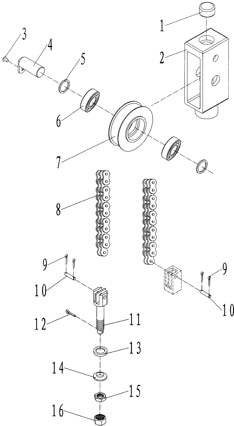
Abbildung 14 Expl. Lastkette
