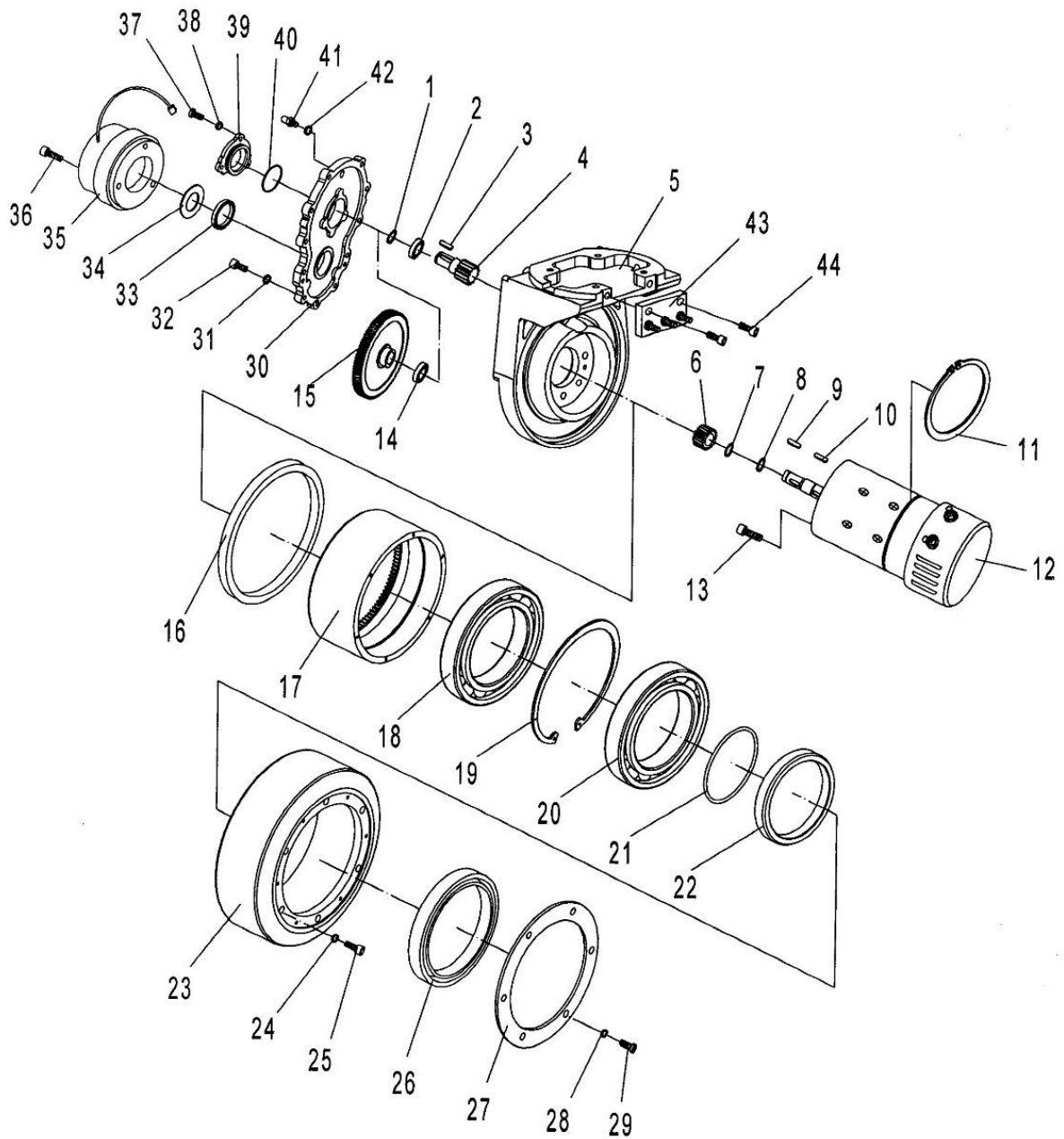
Abbildung 4 Expl. Antriebsrad
