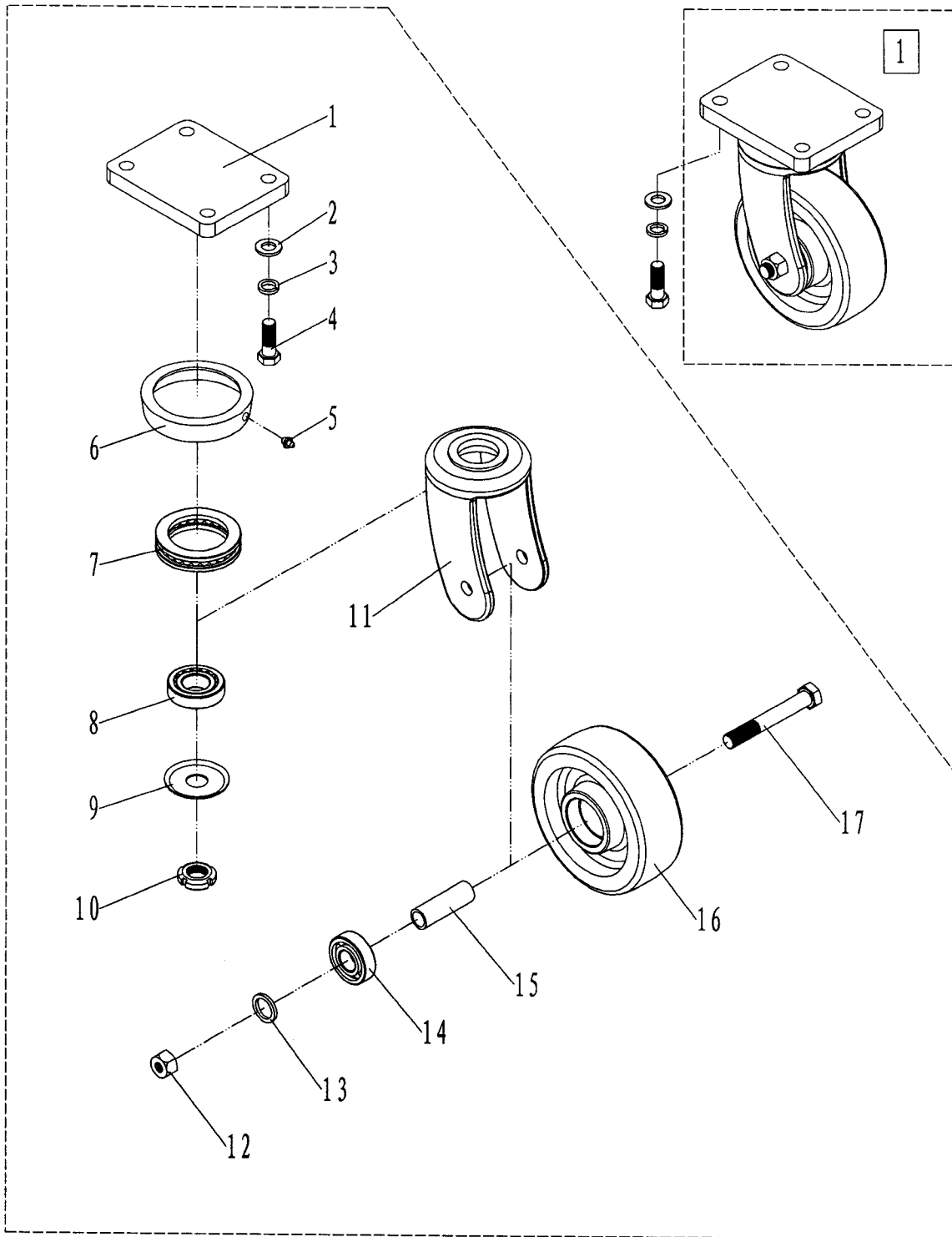
Abbildung 5 Expl. Stützrad
