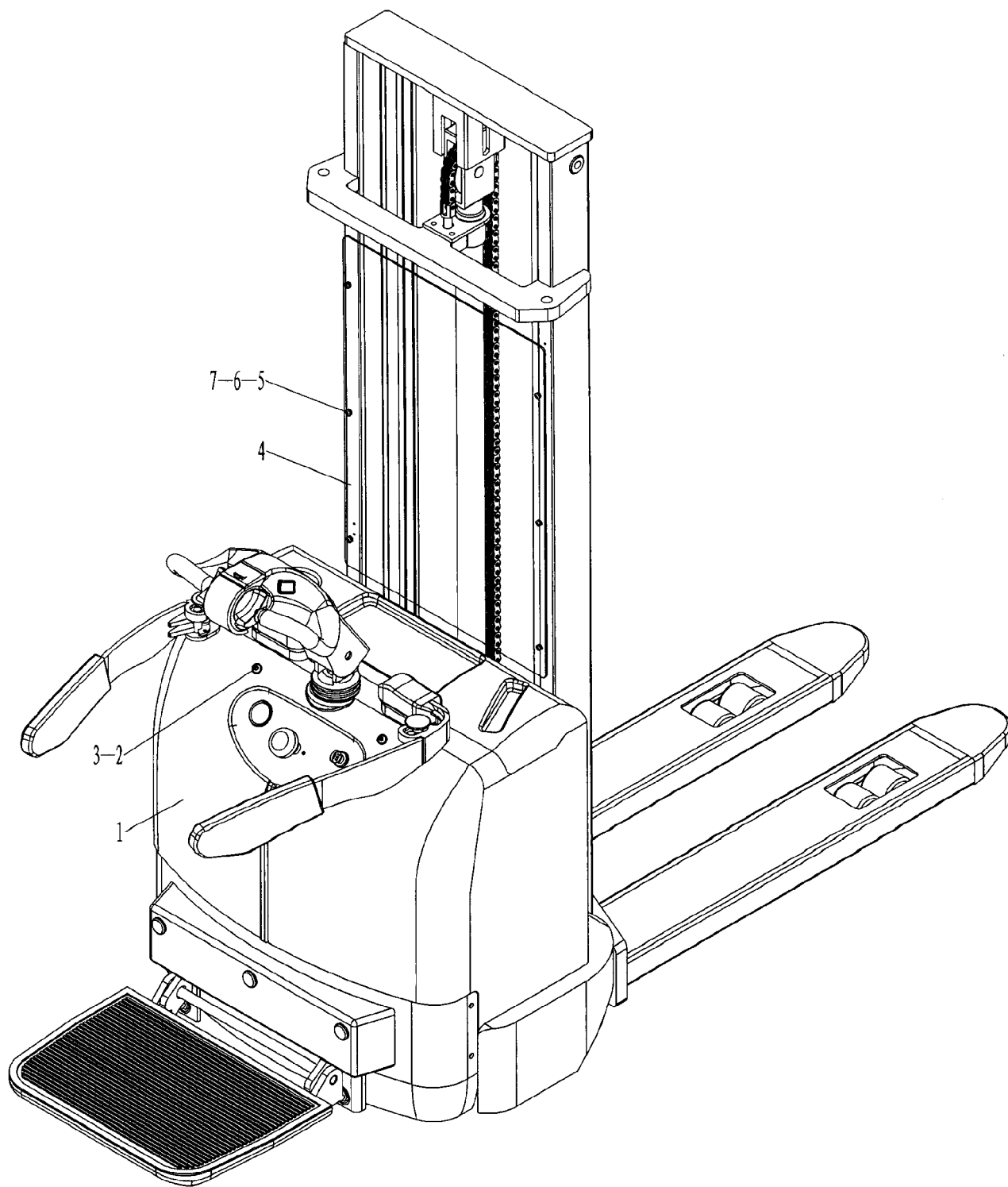
Abbildung 1 Expl. Anbauteil
