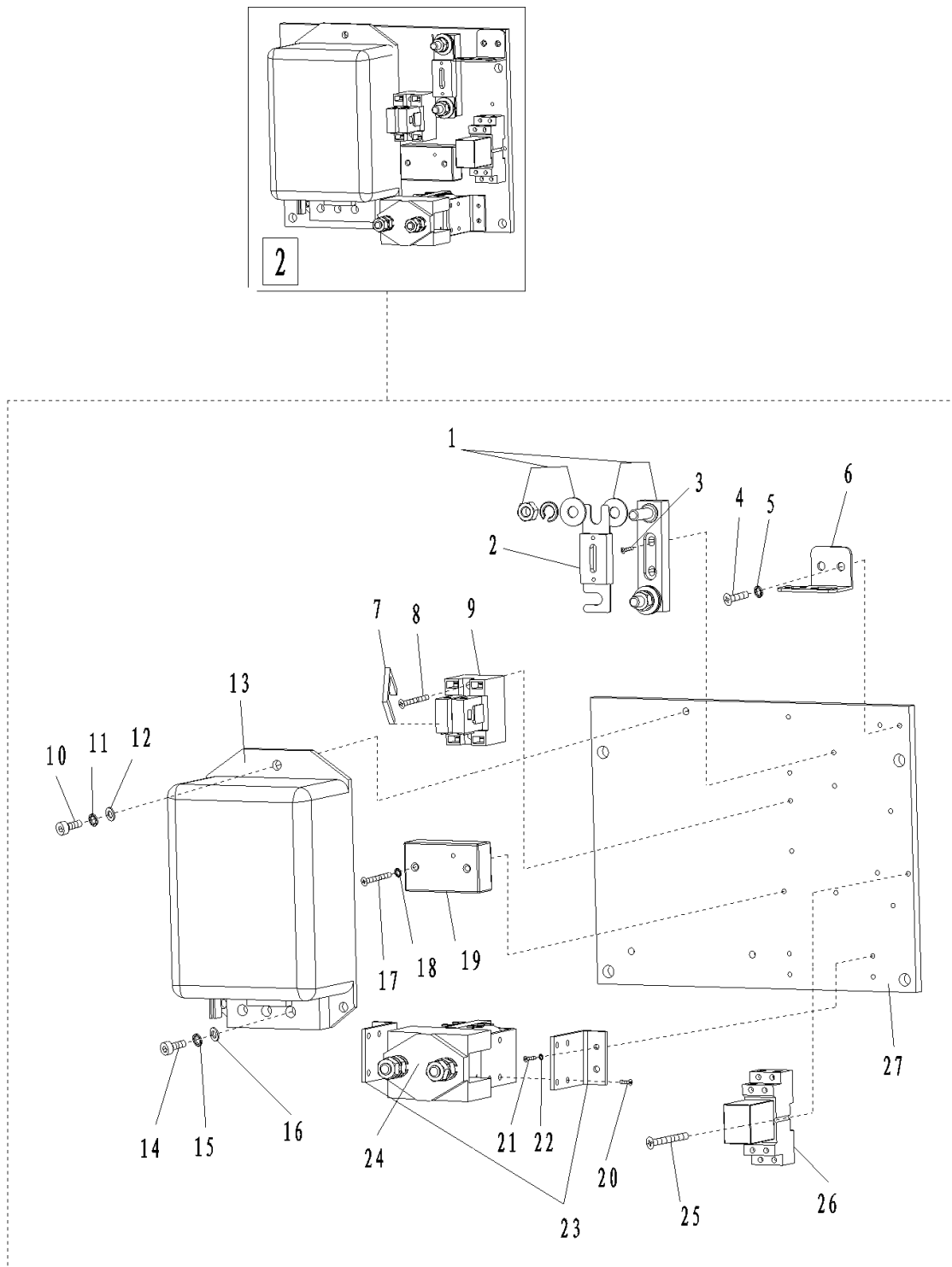
Abbildung 9 Expl. Elektronik
