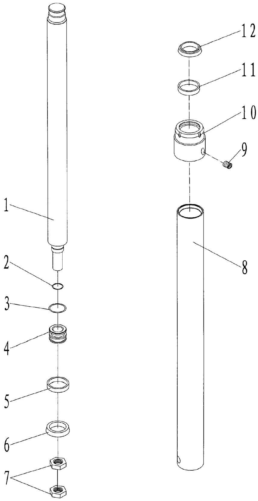
Abbildung 11 Expl. Innerer Hydraulikzylinder
