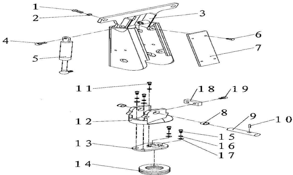
Abbildung 21 Expl. Deichsel
