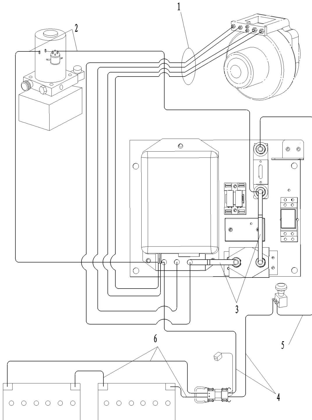
Abbildung 7 Expl. Hauptstromkabel
