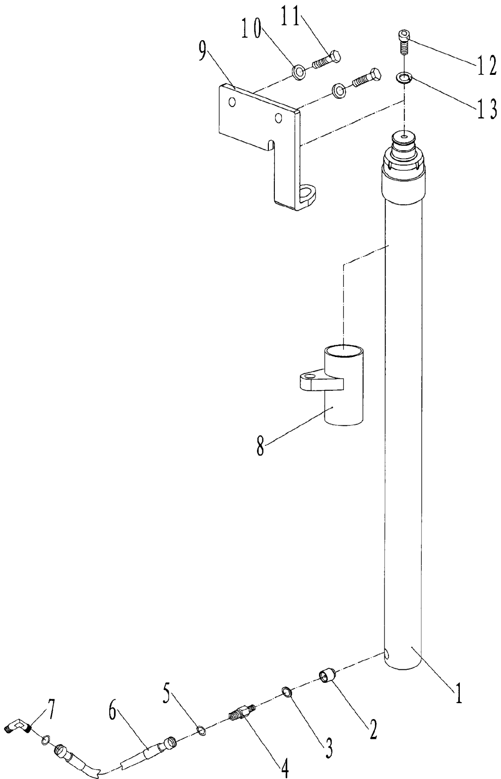
Abbildung 10 Expl. Äußerer Hydraulikzylinder
